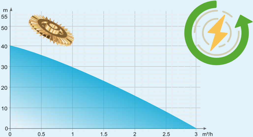
ГРАФІК ЗАЛЕЖНОСТІ ПРОДУКТИВНОСТІ ВІД ТИСКУ
